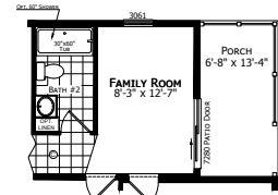
OPTIONAL 1/2 PORCH
