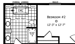
OPTIONAL MASTER BATH
